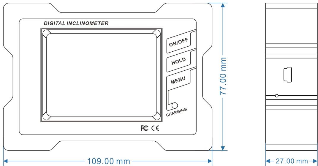
外壳尺寸:L109*H77*W27mm 左侧、底部为强磁吸附面
