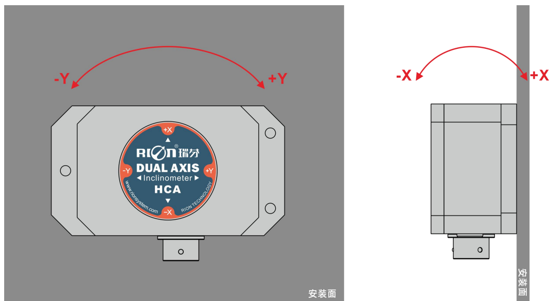
垂直安装
